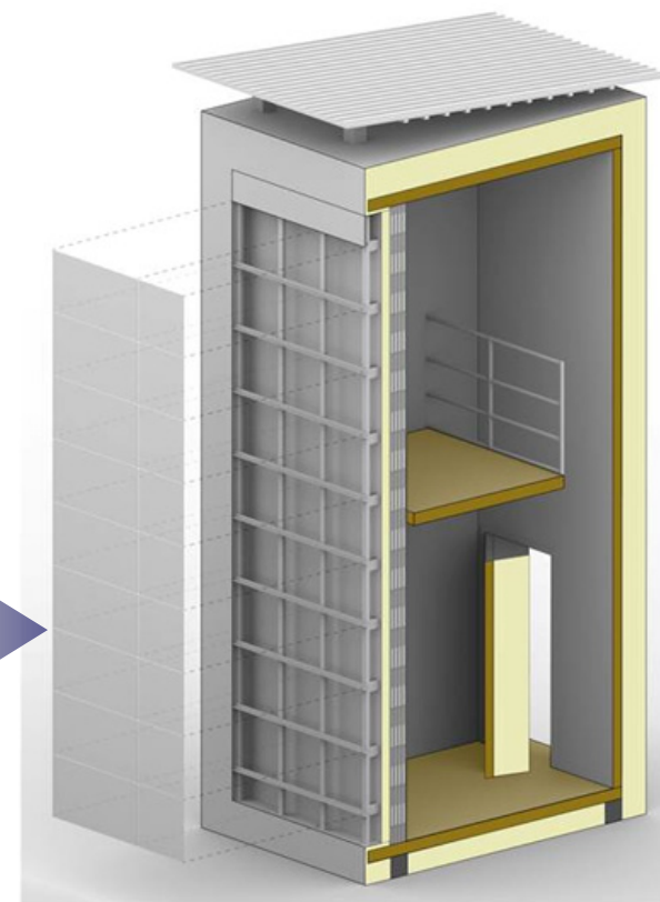
Spaccato assometrico della torretta sperimentale
